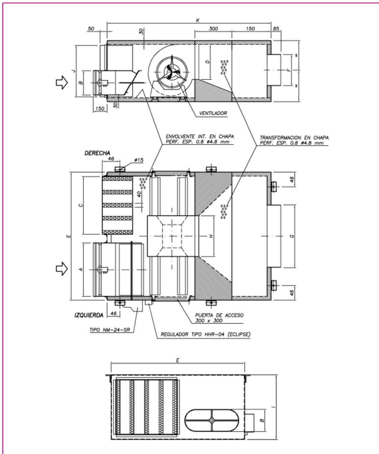
CAJA HVFS 300 a 1500
