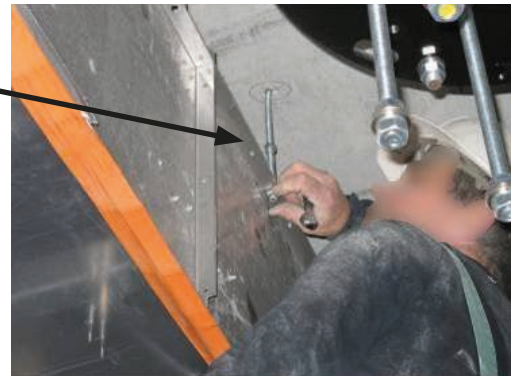
Fijar con arandelas y tuercas
